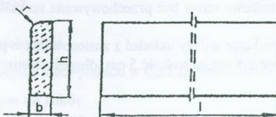
Rysunek 1. Kształt betonowego obrzeża chodnikowego
