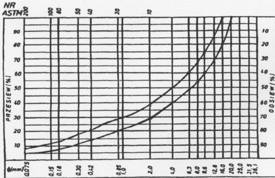
Rys. 4. Krzywe graniczne uziarnienia mieszanki mineralnej 0÷20 mm do warstwy ścierniczej z betonu asfaltowego dla KR 3-6
