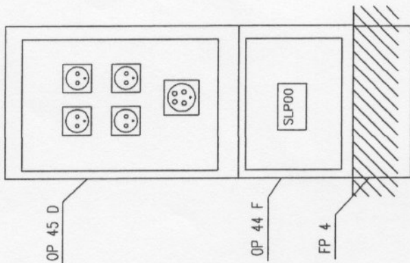
ROZMIESZCZENIE APARATÓW W SKRZYNCY SPE
