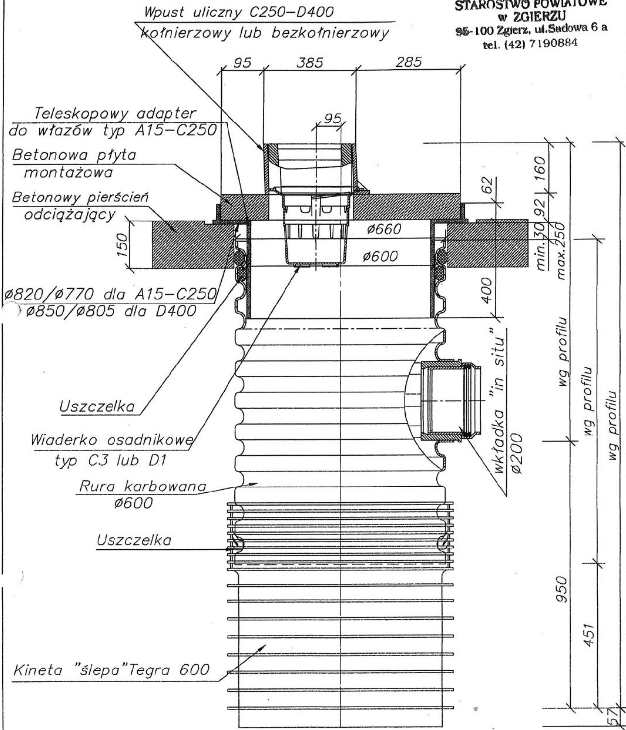
Studzienka deszczowa Tegra 600 z teleskopowym adapterem do włazów i betonowym pierścieniem odcciążającym oraz wpustem ulicznym klasy C250-D400
