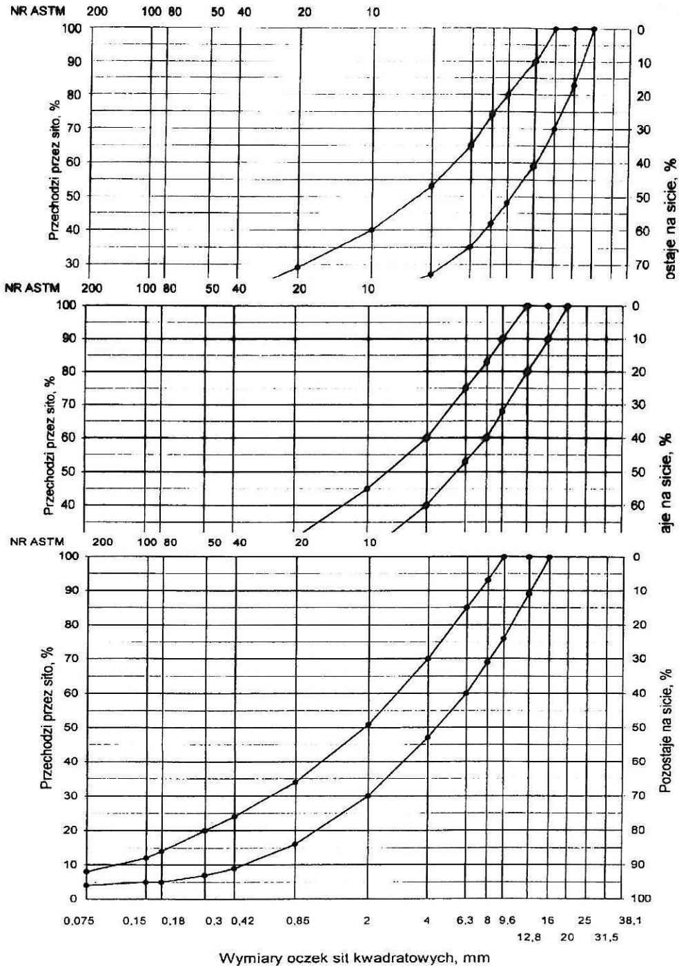
Rys. 5. Krzywe graniczne uziarnienia mieszanki mineralnej BA od 0 do 12,8 mm do podbudowy nawierzchni drogi o obciążeniu ruchem KR 1 lub KR 2
