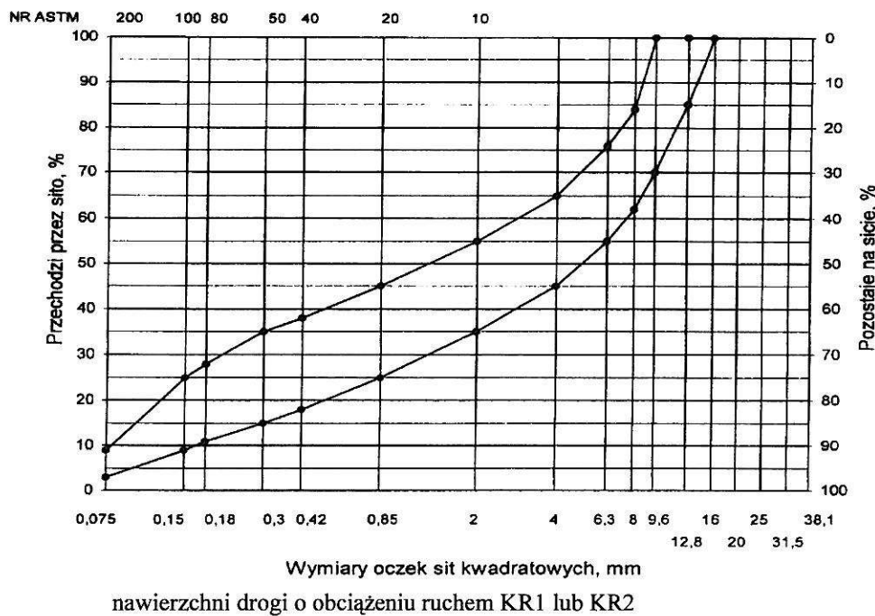
Rys. 10. Krzywe graniczne uziarnienia mieszanki mineralnej BA od 0 do 12,8 mm do warstwy wiążącej, wyrównawczej i wzmacniającej
