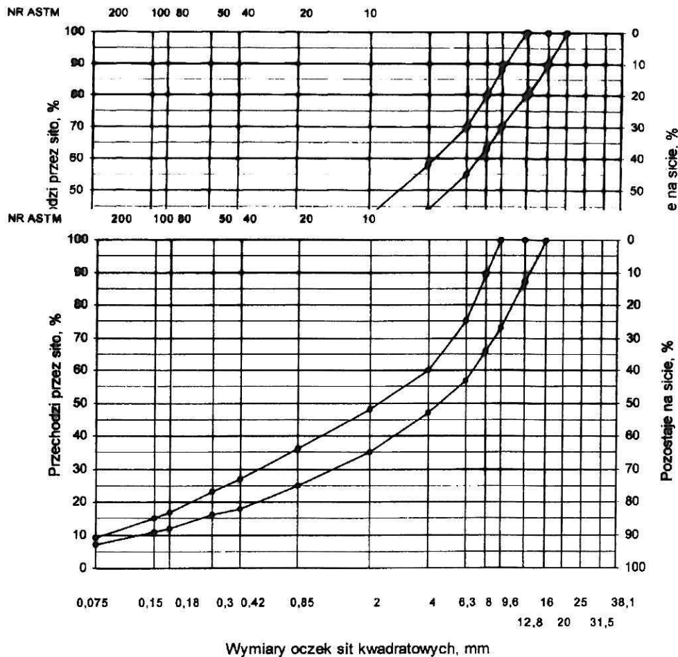
Rys. 7. Krzywe graniczne uziarnienia mieszanki mineralnej BA od 0 do 12,8 mm do warstwy ścieralnej nawierzchni drogi o obciążeniu ruchem od KR3 do KR6
