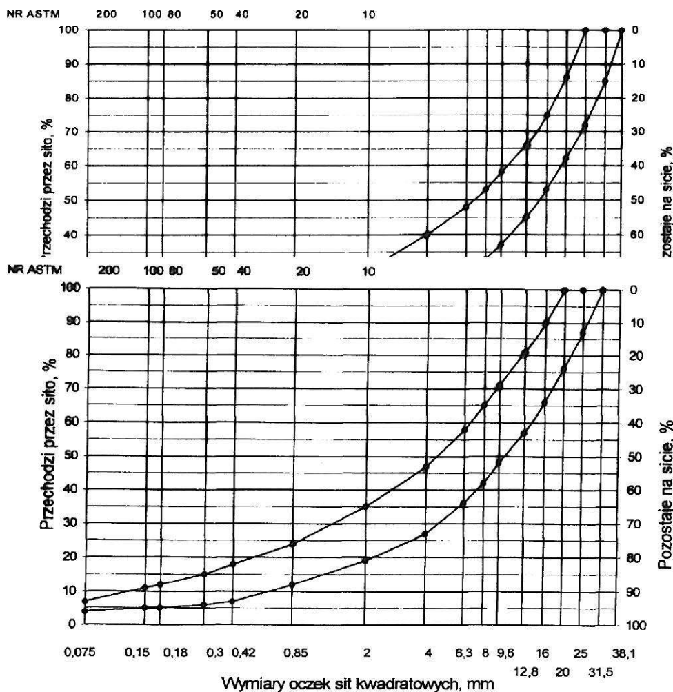
Rys. 6. Krzywe graniczne uziarnienia mieszanki mineralnej BA od 0 do 31,5 mm podbudowy nawierzchni drogi o obciążeniu ruchem od KR 3 do KR 6
