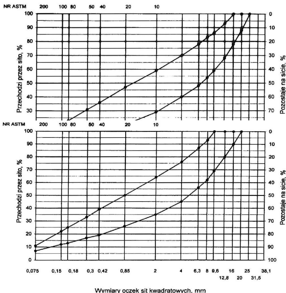
Rys. 1. Krzywe graniczne uziarnienia mieszanki mineralnej BA od 0 do 20 mm do warstwy ścieralnej nawierzchni drogi o obciążeniu ruchem dla KR1 lub KR2
