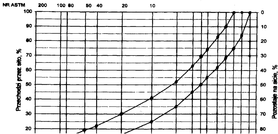
Rys. 11. Krzywe graniczne uziarnienia mieszanki mineralnej BA od 0 do 25 mm do warstwy wiążącej, wyrównawczej i wzmacniającej nawierzchni drogi o obciążeniu ruchem od KR3 do KR6
