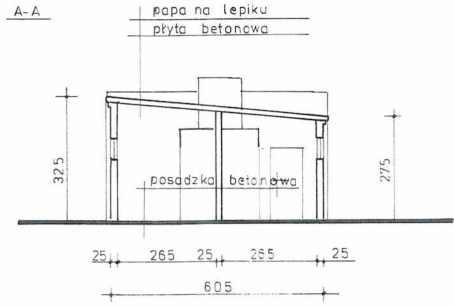
PRZEKRÓJ
